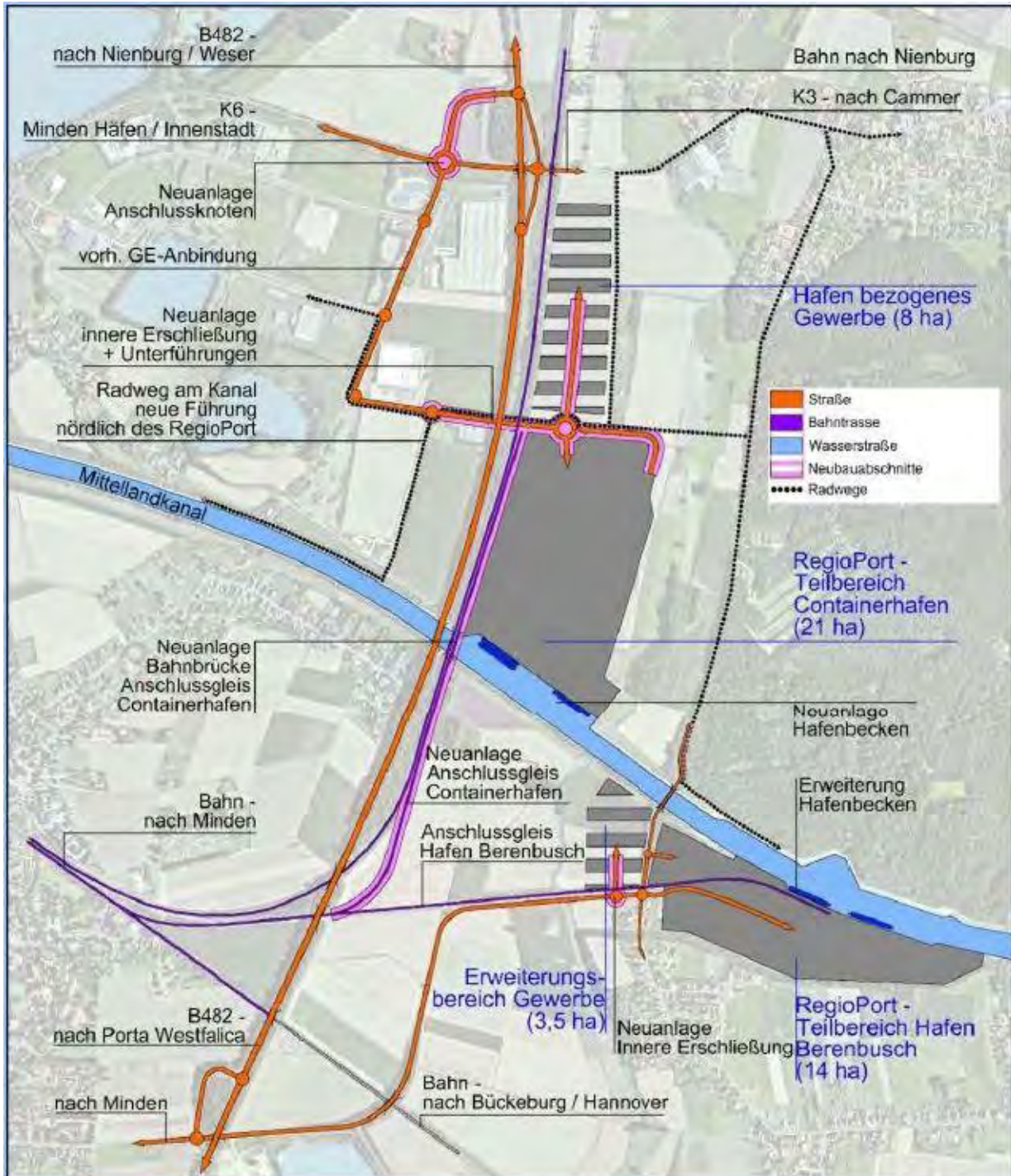
Karte: Strukturplan zum RegioPort Minden; nicht vollständig aktuell; ein aktualisierter Strukturplan liegt uns nicht vor.
