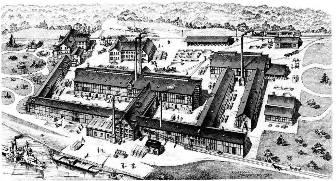
Plan: Dampfziegelei Heisterholz, F. Schütte, Heisterholz a. d. Weser, Anno 1910.
