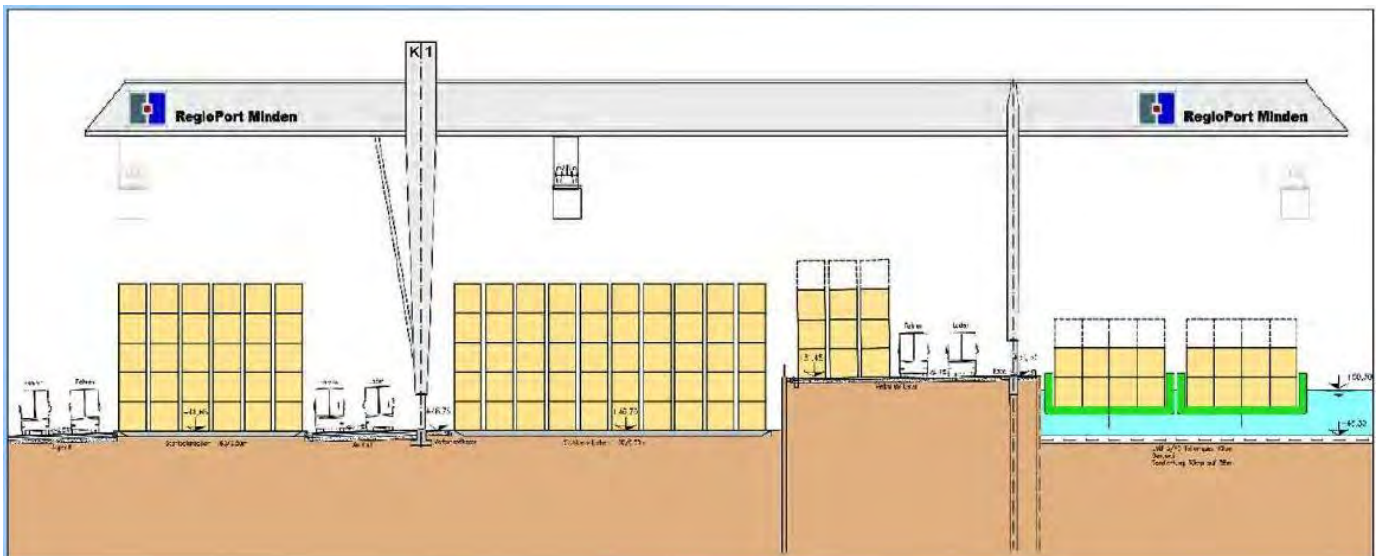
Grafik: Schnitt Anlegestelle Umschlag im RegioPort Minden.
