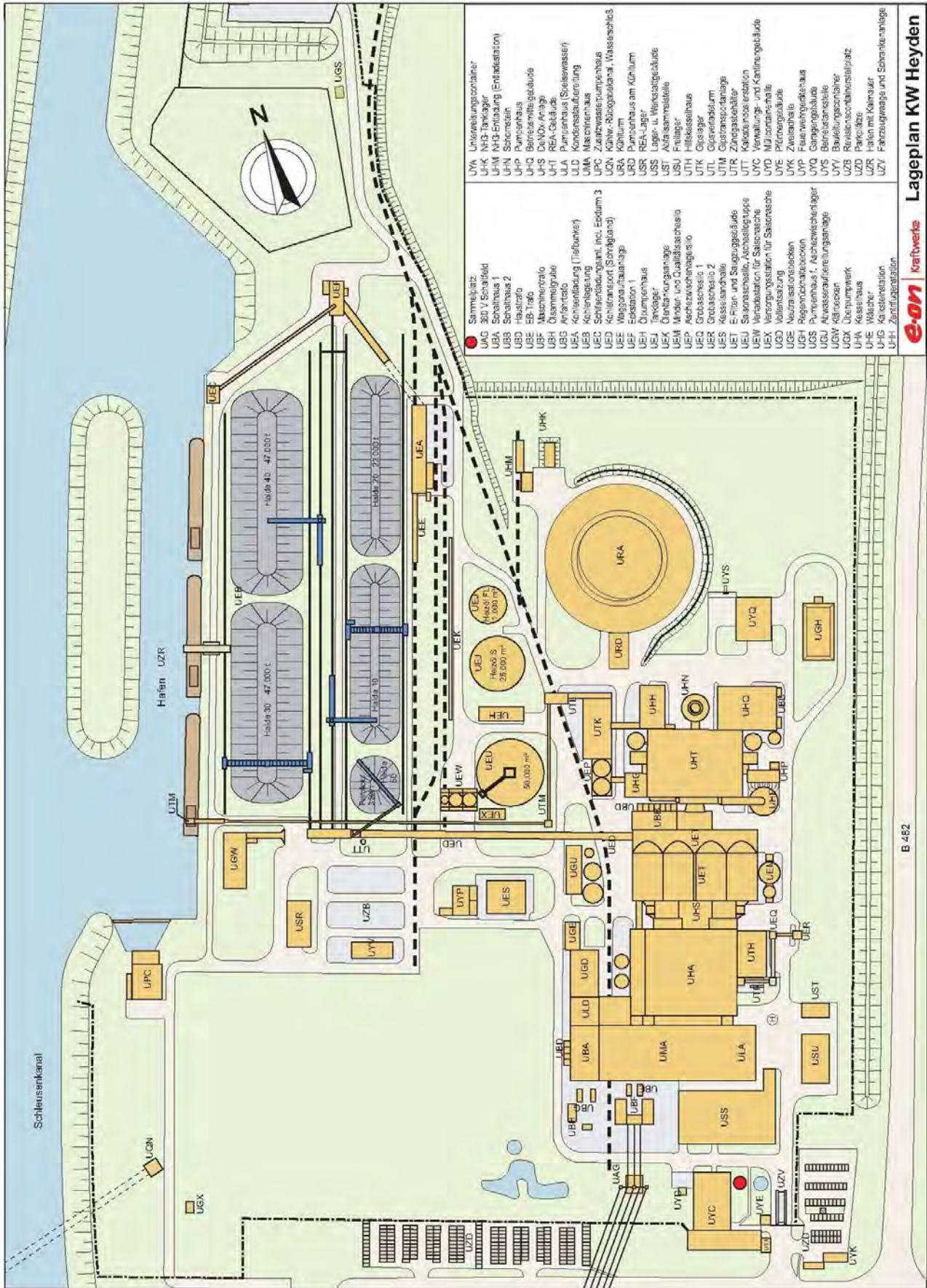
Plan: Lageplan des Kraftwerks Heyden in Petershagen-Lahde.
