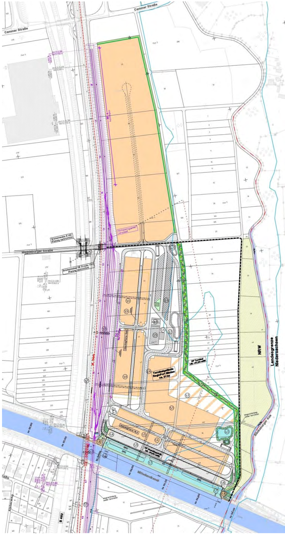
Karte: Übersichtslageplan RegioPort Minden.
