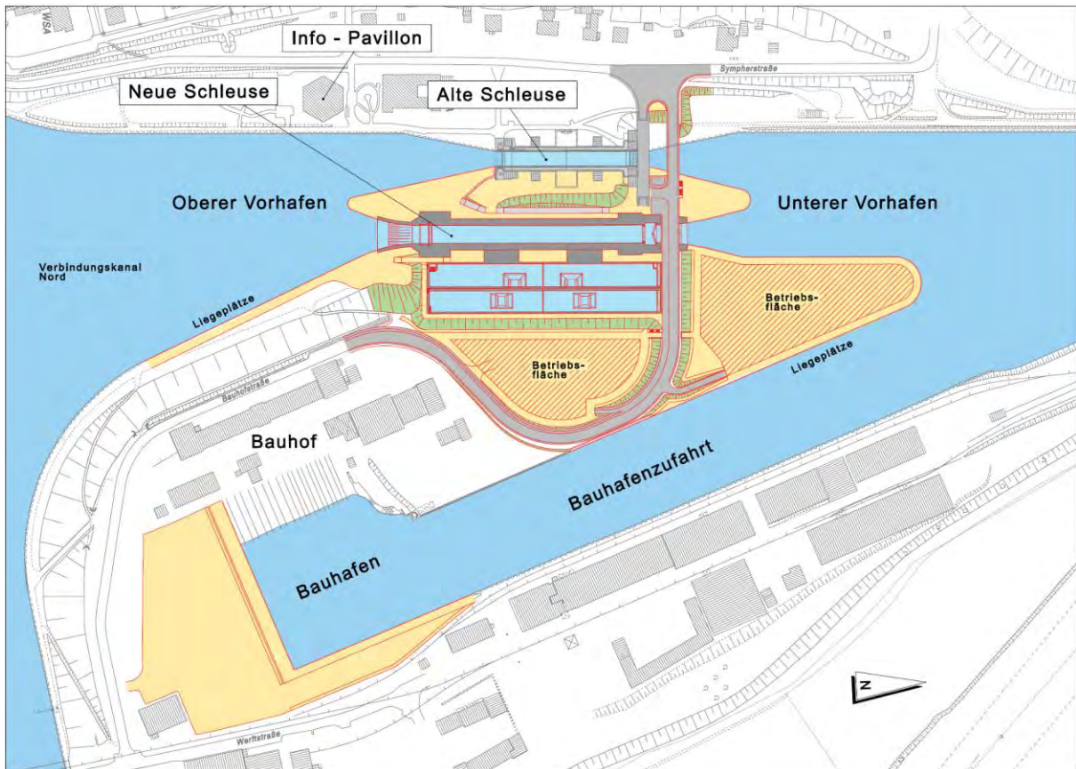
Plan: Neue und alte Schleuse in Minden.
