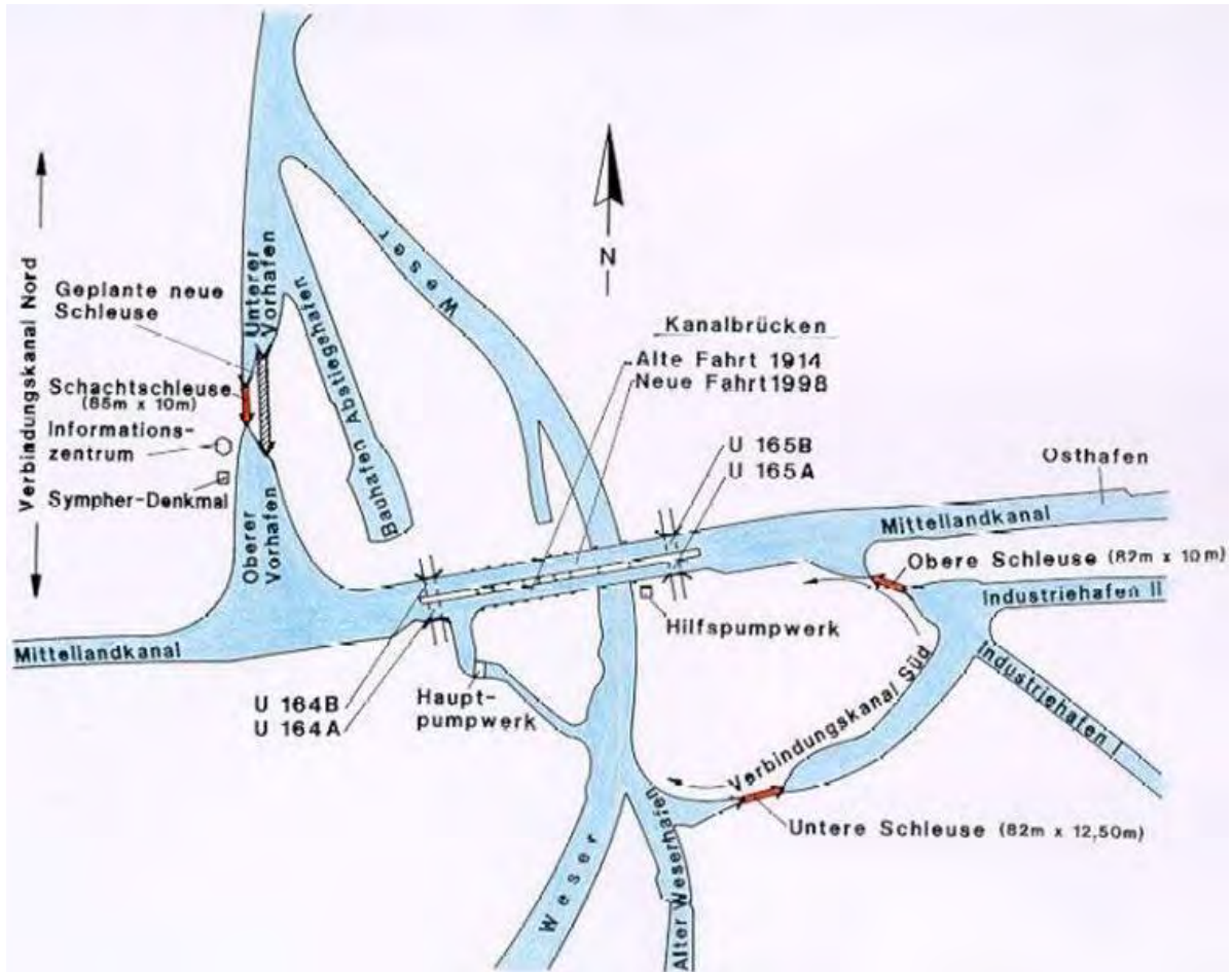
Karte: Der Bereich um das Wasserstraßenkreuz Minden.
