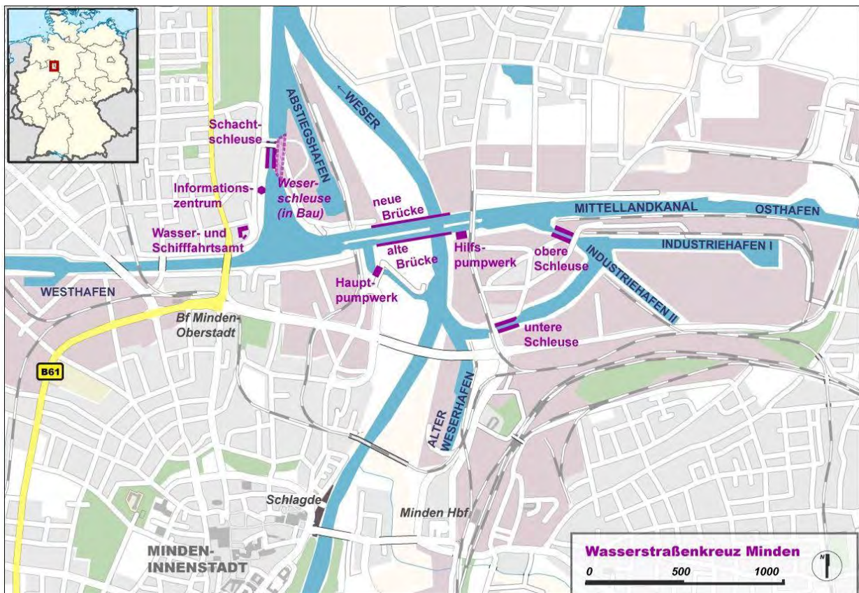
Karte: Der Bereich um das Wasserstraßenkreuz Minden.
